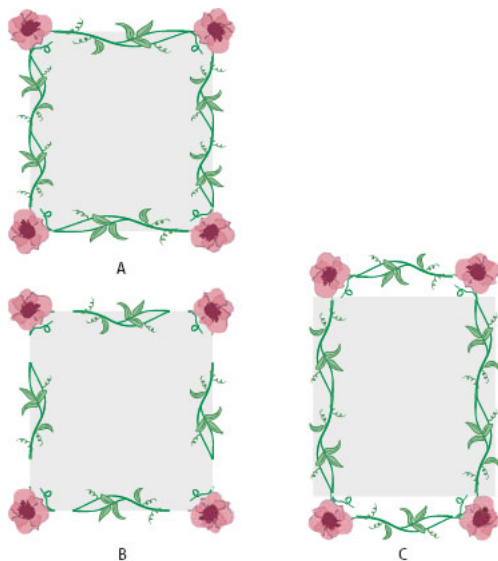
Fit options
